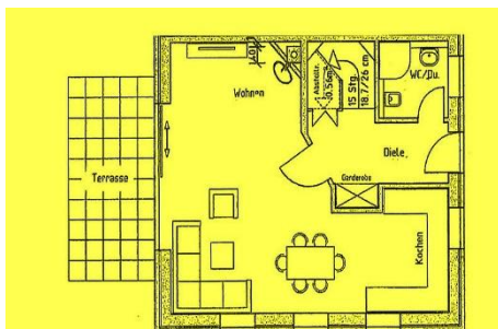
Grundriss EG
